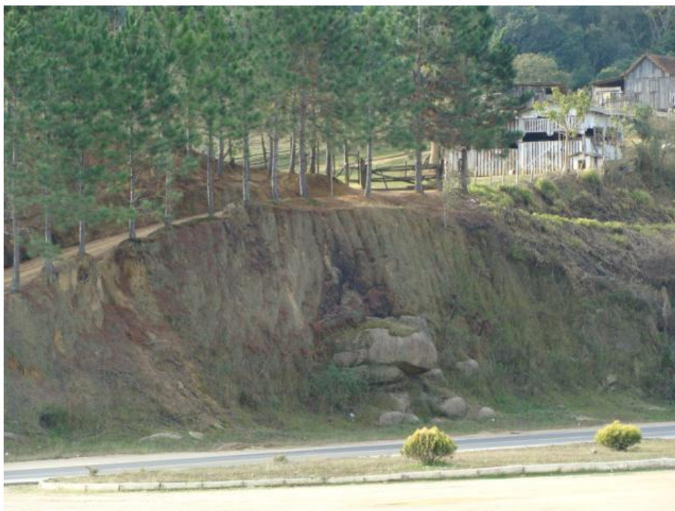
Figura 11 - Afloramento do aquífero fraturado de litologia granítica ampliado por espessa zona
