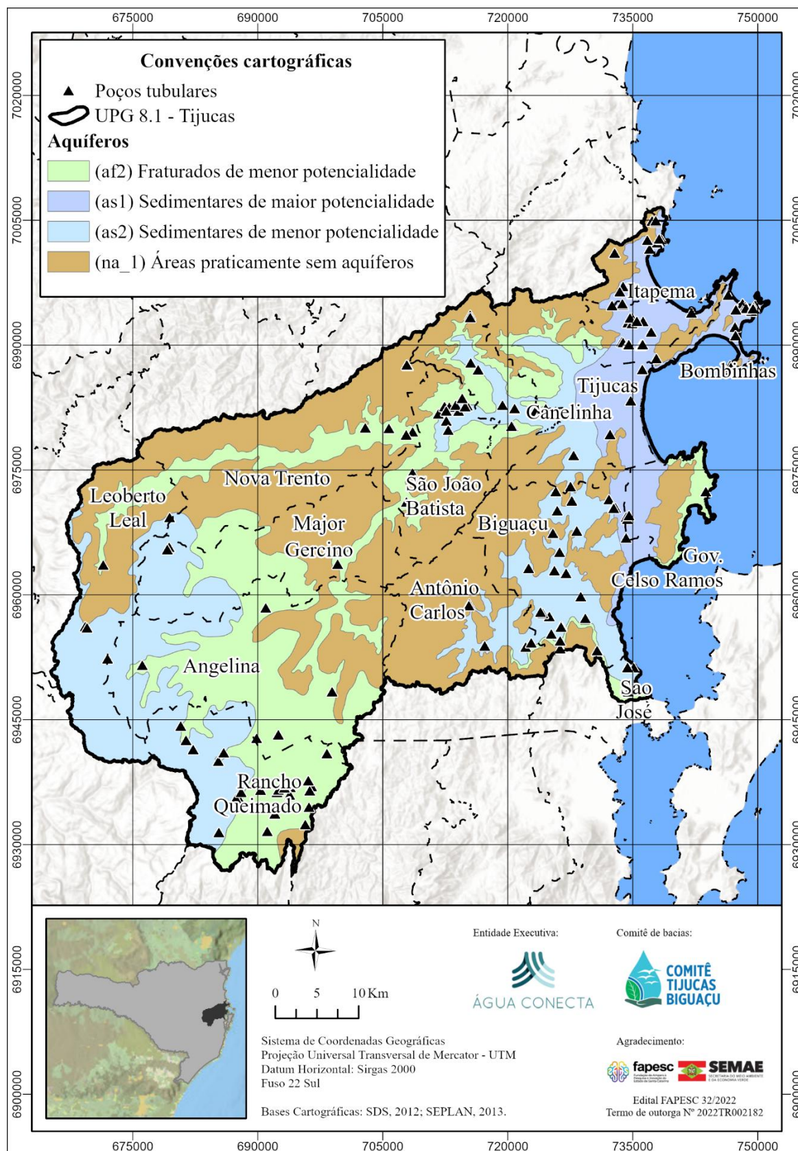
Figura 37 - Mapa das Zonas Aquíferas da UPG 8.1 – Tijucas e localização dos poços cadastrados no SIAGAS, CNARH e SIOUT.
