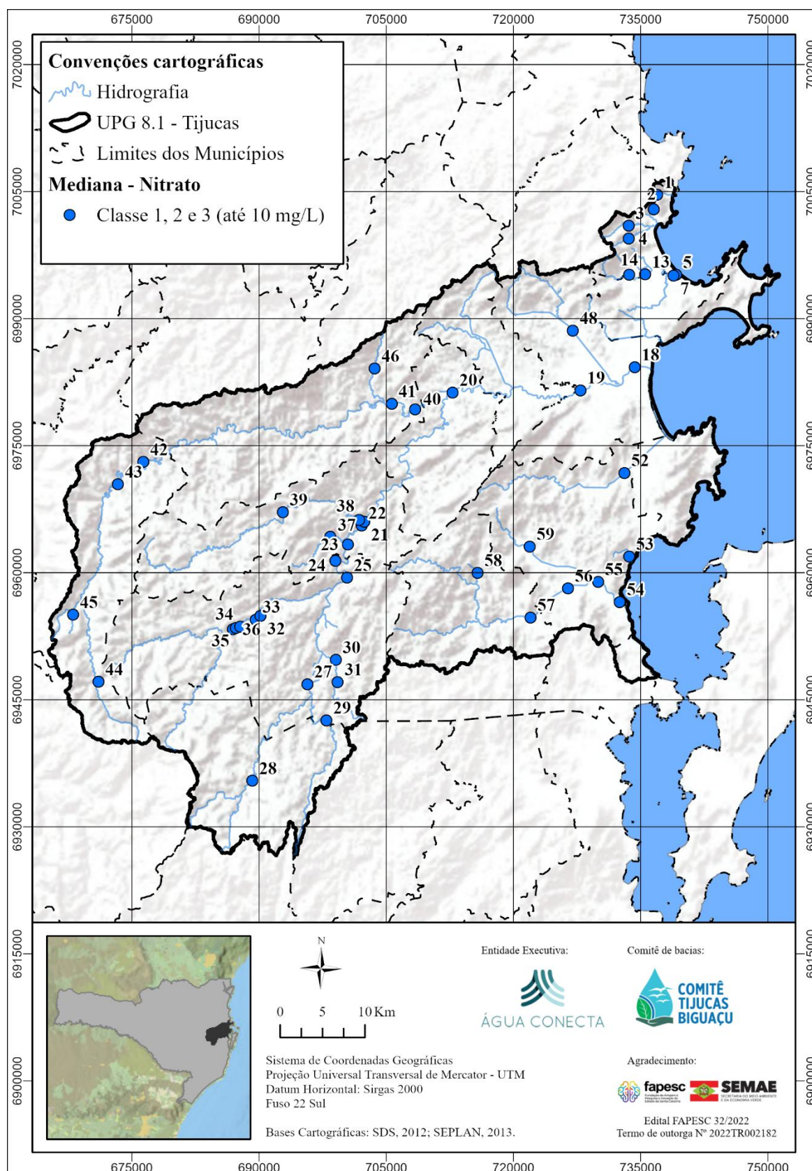
Figura 26 - Síntese dos dados da situação atual de nitrato ( \text{NO}_3^- ) na UPG 8.1 – Tijucas
