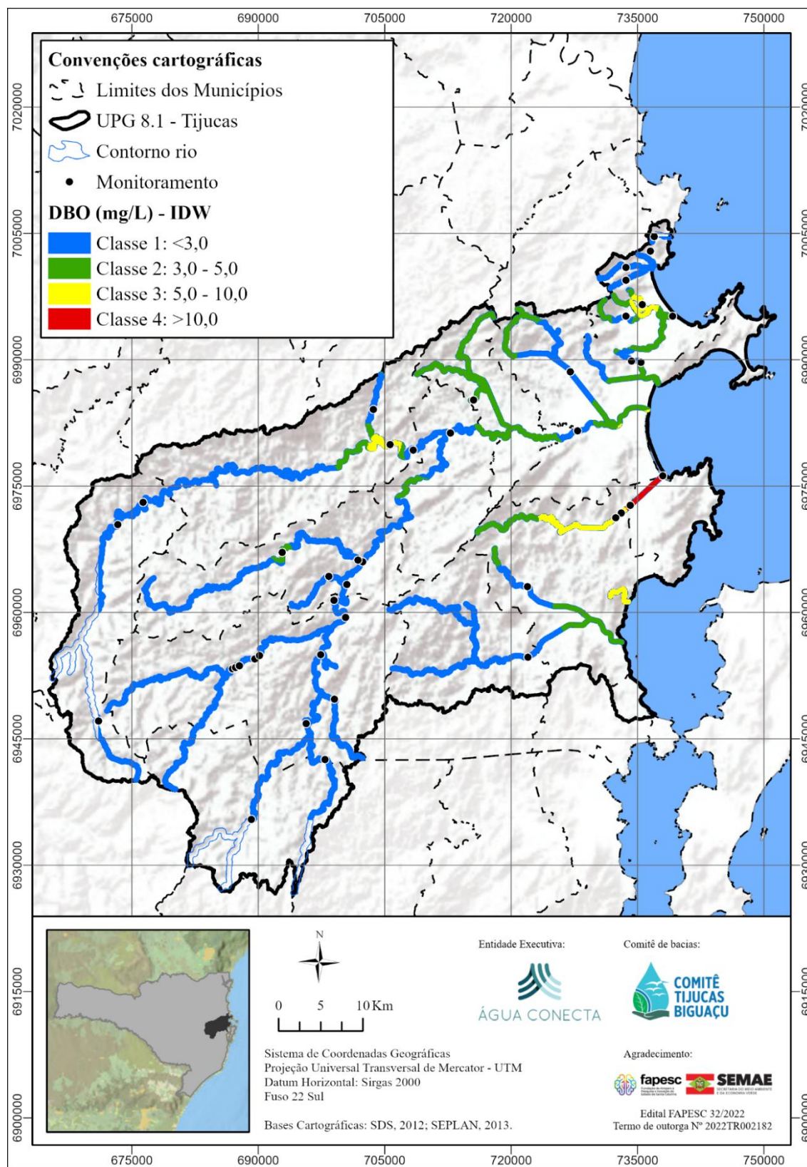
Figura 30 - Interpolação (IDW) das concentrações de DBO nos pontos de monitoramento da UPG 8.1 – Tijucas
