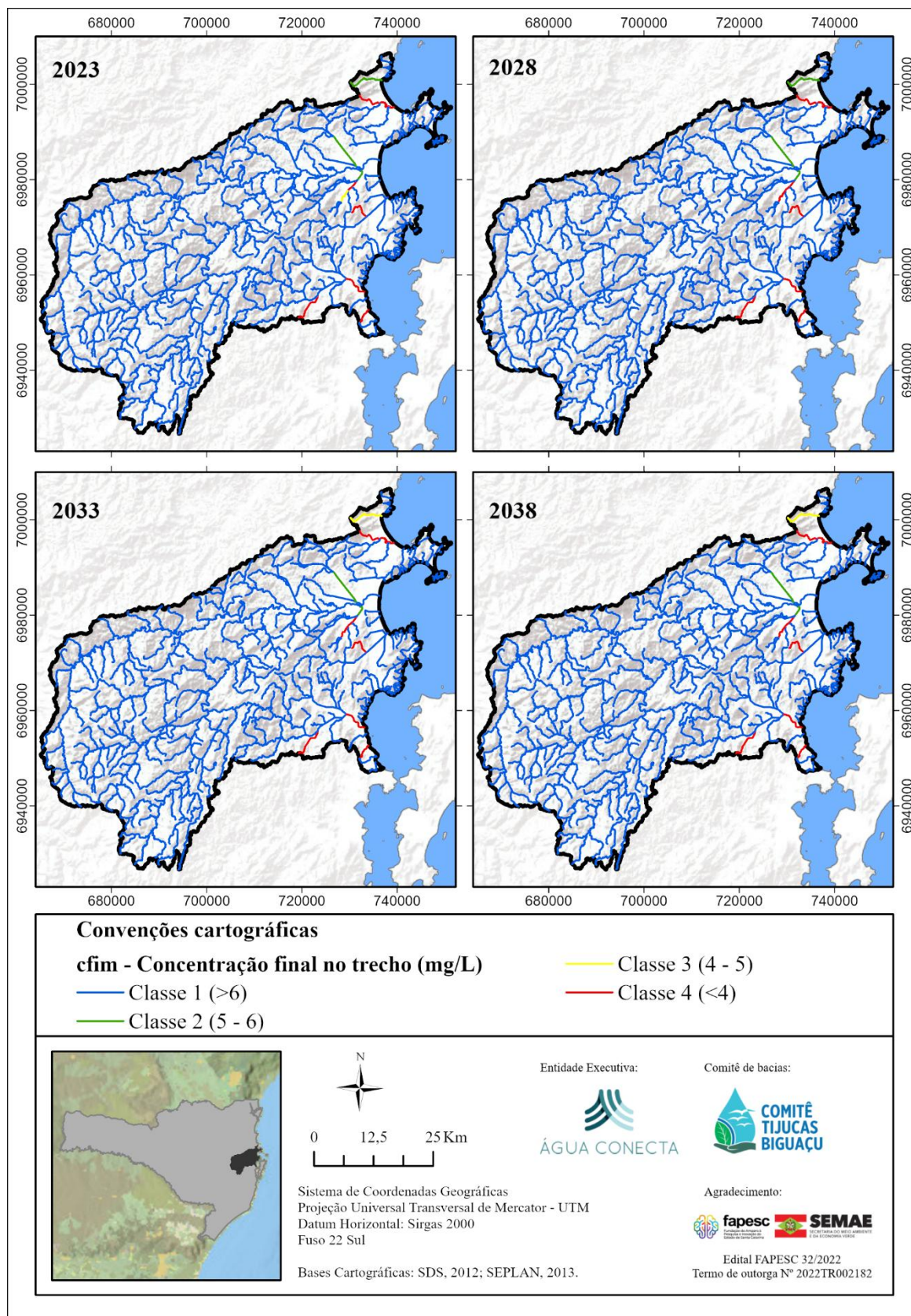
Figura 61 – Cenário atual (2023) e otimista para os horizontes curto (2028), médio (2033) e longo (2038) prazo para a OD, dezembro (Tijucas) e janeiro (Biguaçu) de 2023.
