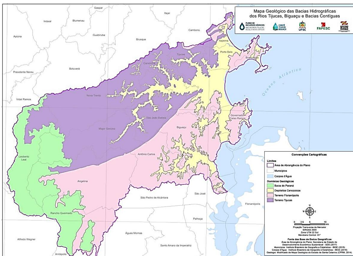
Figura 9 - Mapa Geológico dos Domínios presentes nas bacias hidrográficas dos Rios Tijucas, Biguaçu e bacias contíguas
