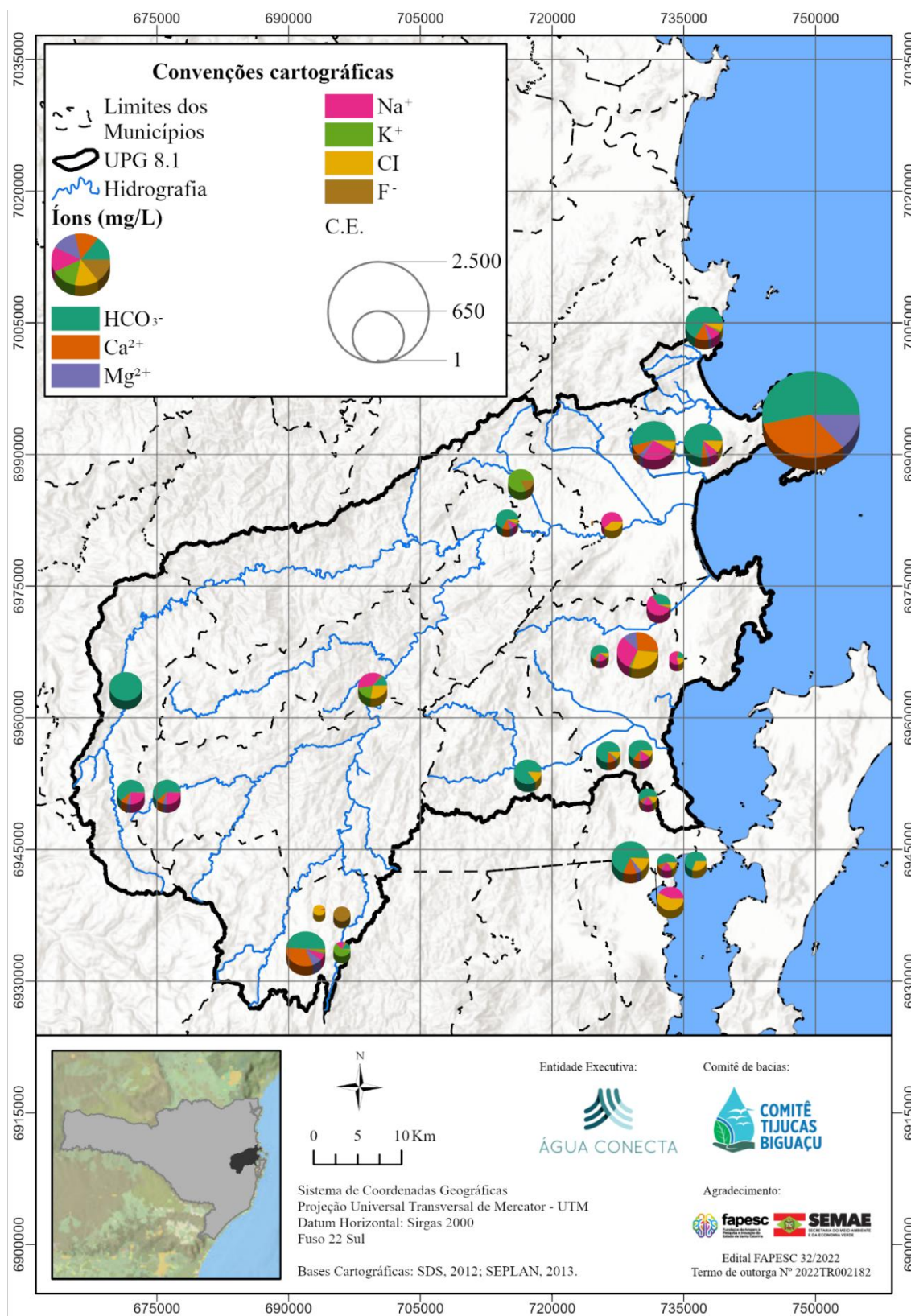
Figura 39 – Distribuição da composição iônica (íons maiores) das águas subterrâneas na UPG 8.1 - Tijucas. Os diâmetros dos gráficos indicam a ionização total das amostras (condutividade elétrica).
