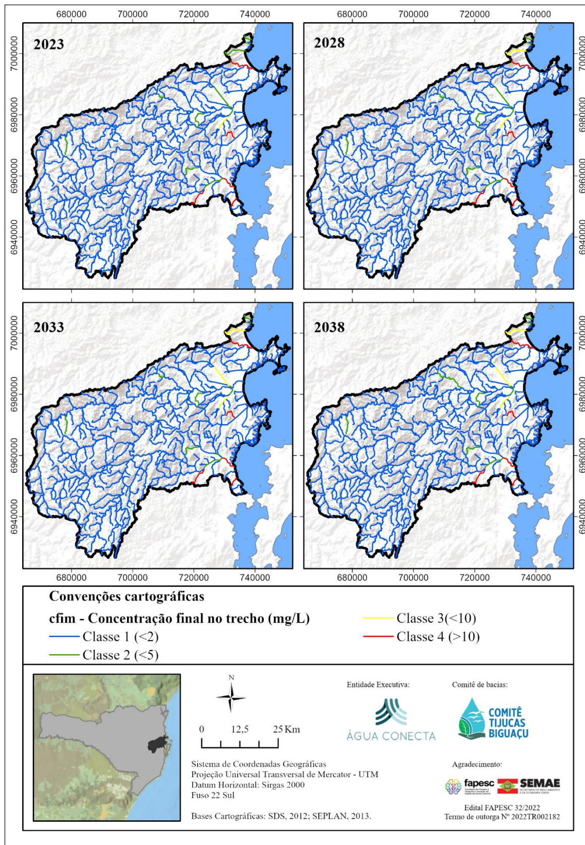
Figura 58 – Cenário atual (2023) e otimista para os horizontes curto (2028), médio (2033) e longo (2038) prazo para a DBO 5,20 , dezembro (Tijucas) e janeiro (Biguaçu) de 2023.
