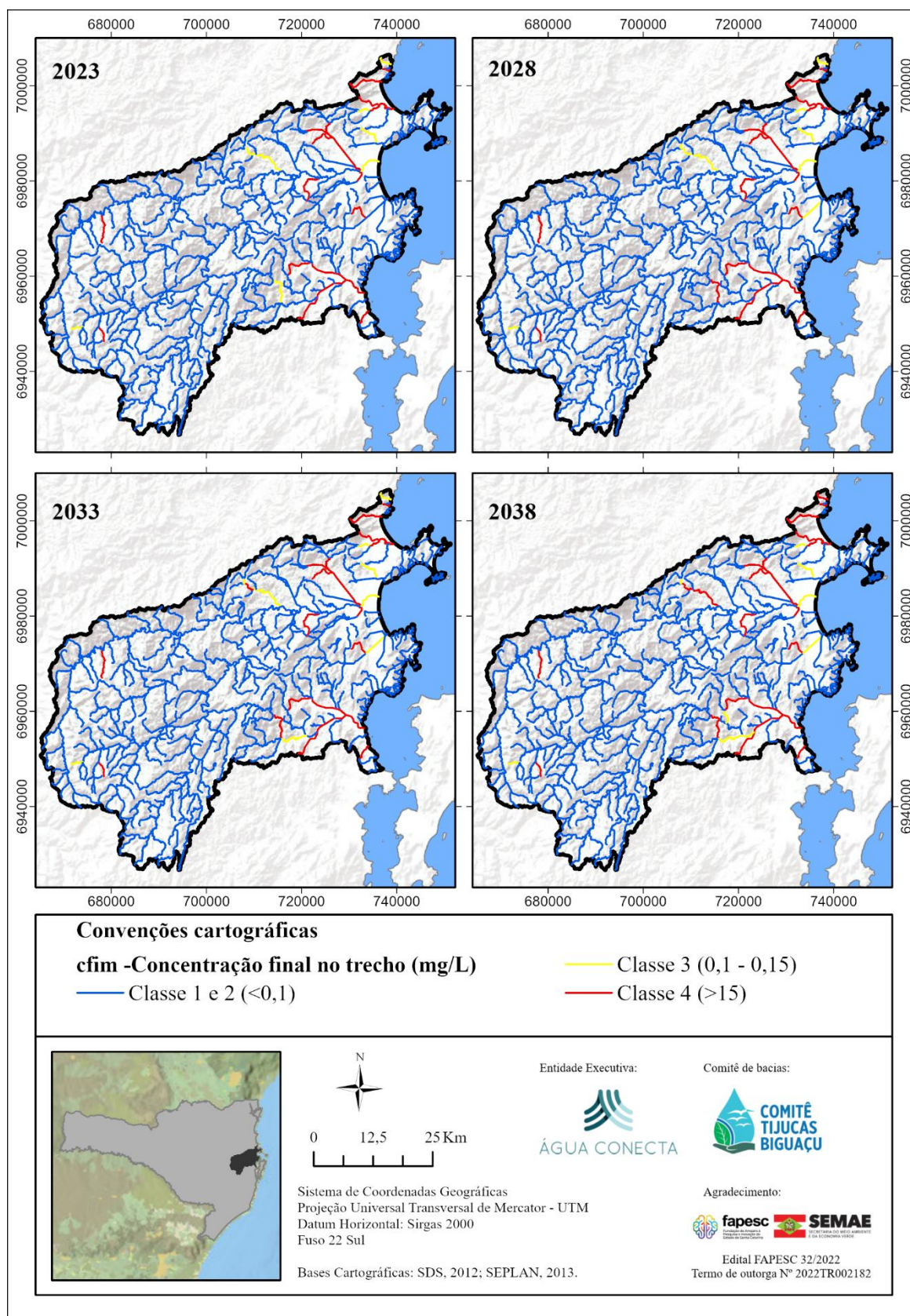
Figura 62 – Cenário atual (2023) e tendencial para os horizontes curto (2028), médio (2033) e longo (2038) prazo para a Pt, dezembro (Tijucas) e janeiro (Biguaçu) de 2023.
