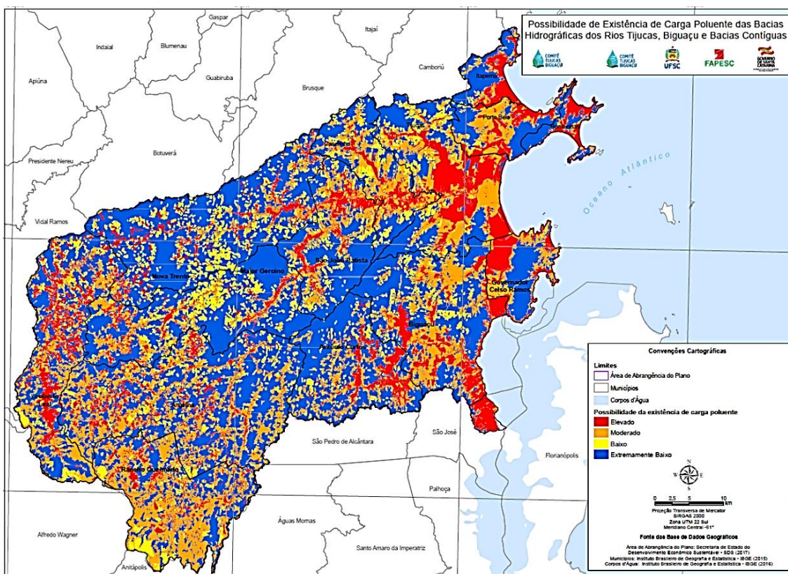
Figura 48 - Mapa de possibilidade da existência de carga poluente
