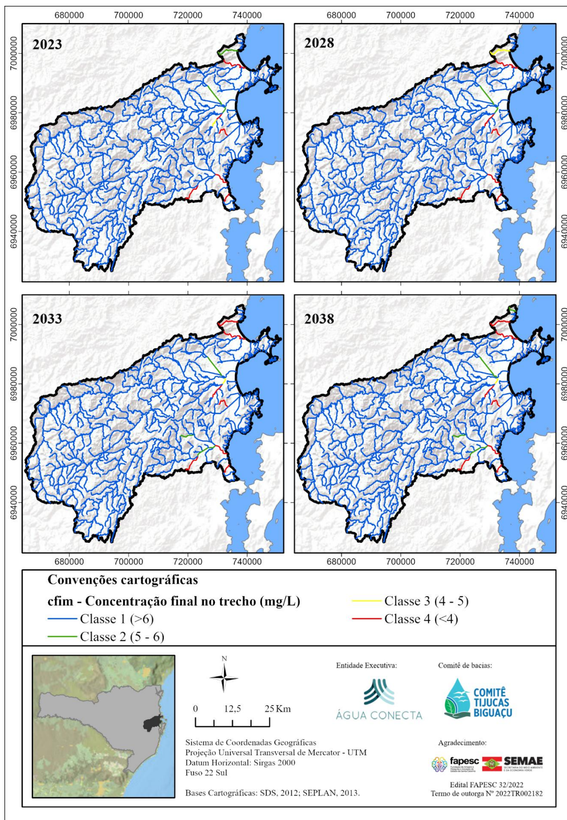
Figura 60 – Cenário atual (2023) e crítico para os horizontes curto (2028), médio (2033) e longo (2038) prazo para a OD
