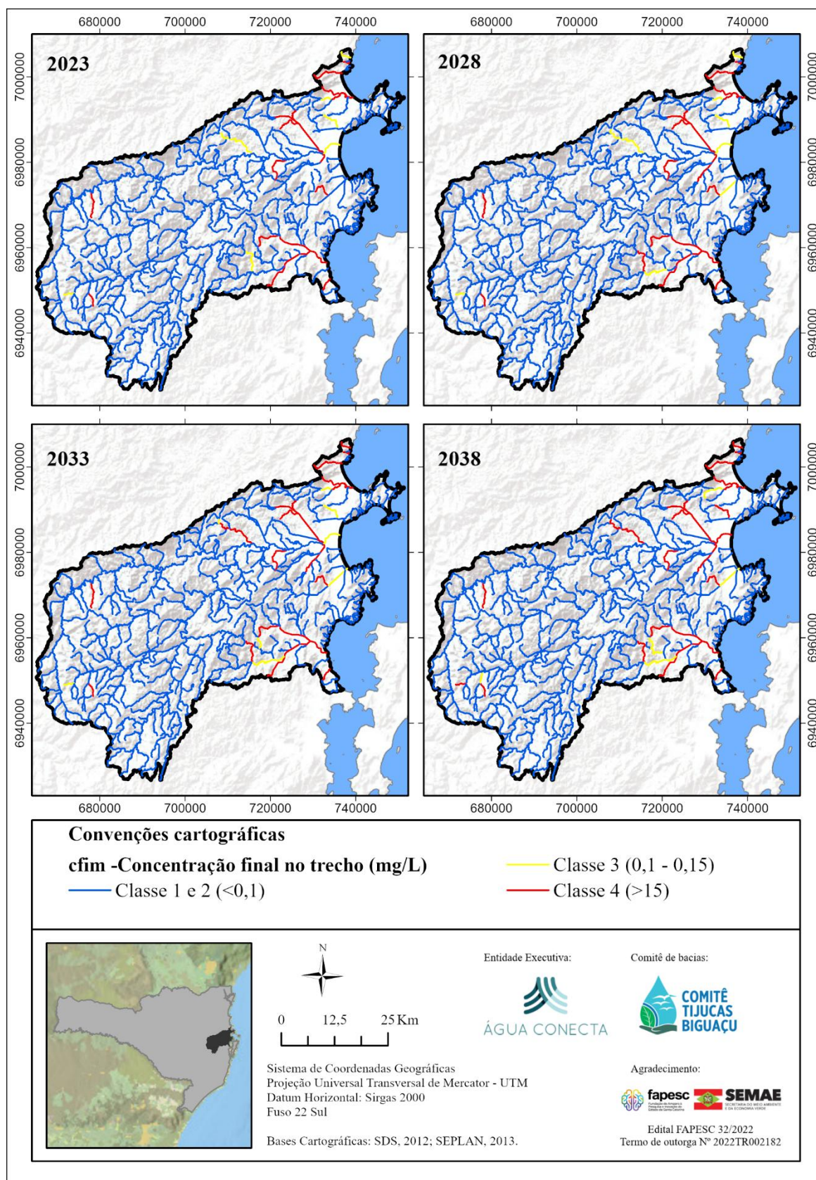
Figura 63 – Cenário atual (2023) e crítico para os horizontes curto (2028), médio (2033) e longo (2038) prazo para a Pt, dezembro (Tijucas) e janeiro (Biguaçu) de 2023.
