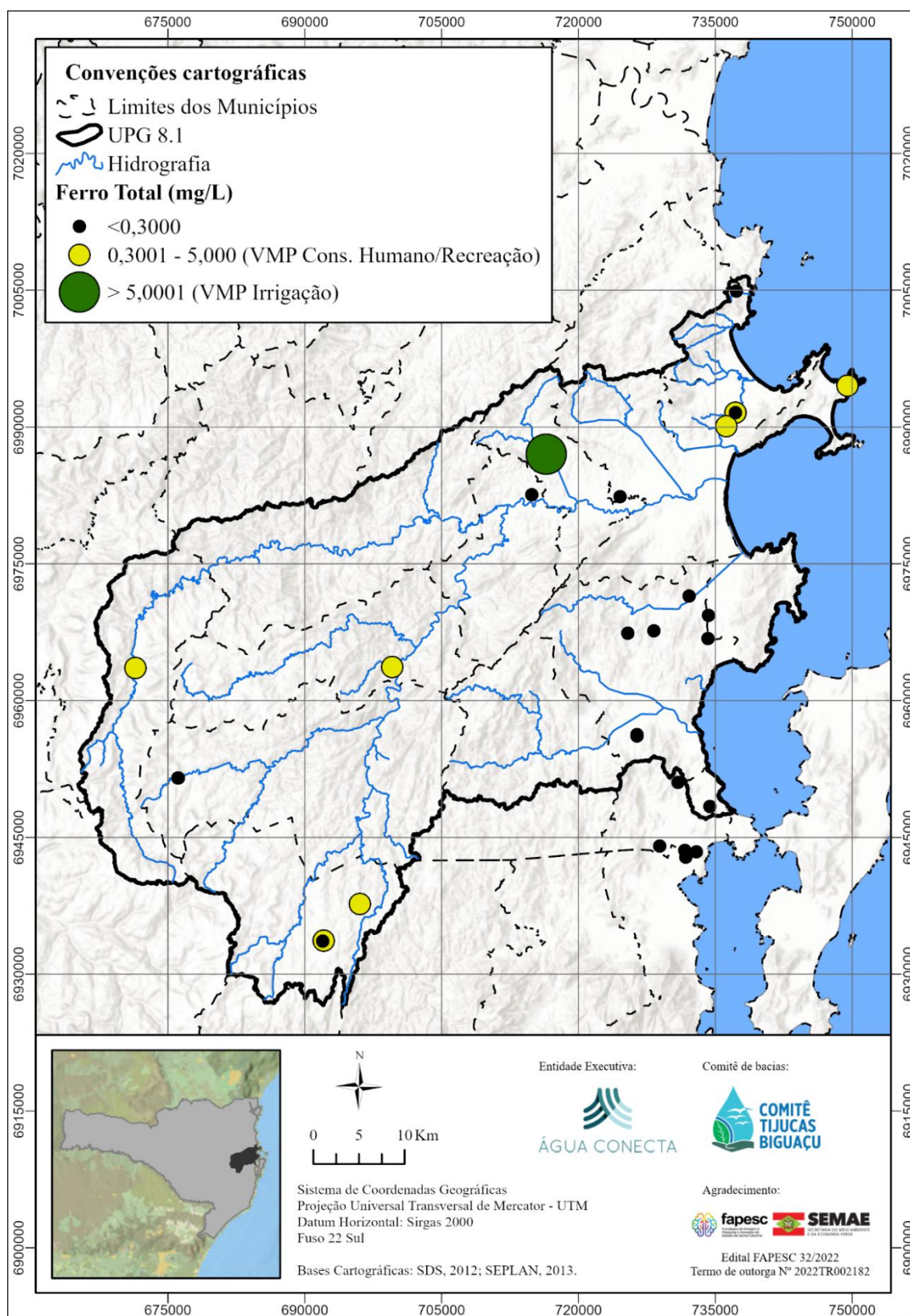
Figura 42 - Distribuição da concentração de ferro nas águas subterrâneas da UPG 8.1 – Tijucas
