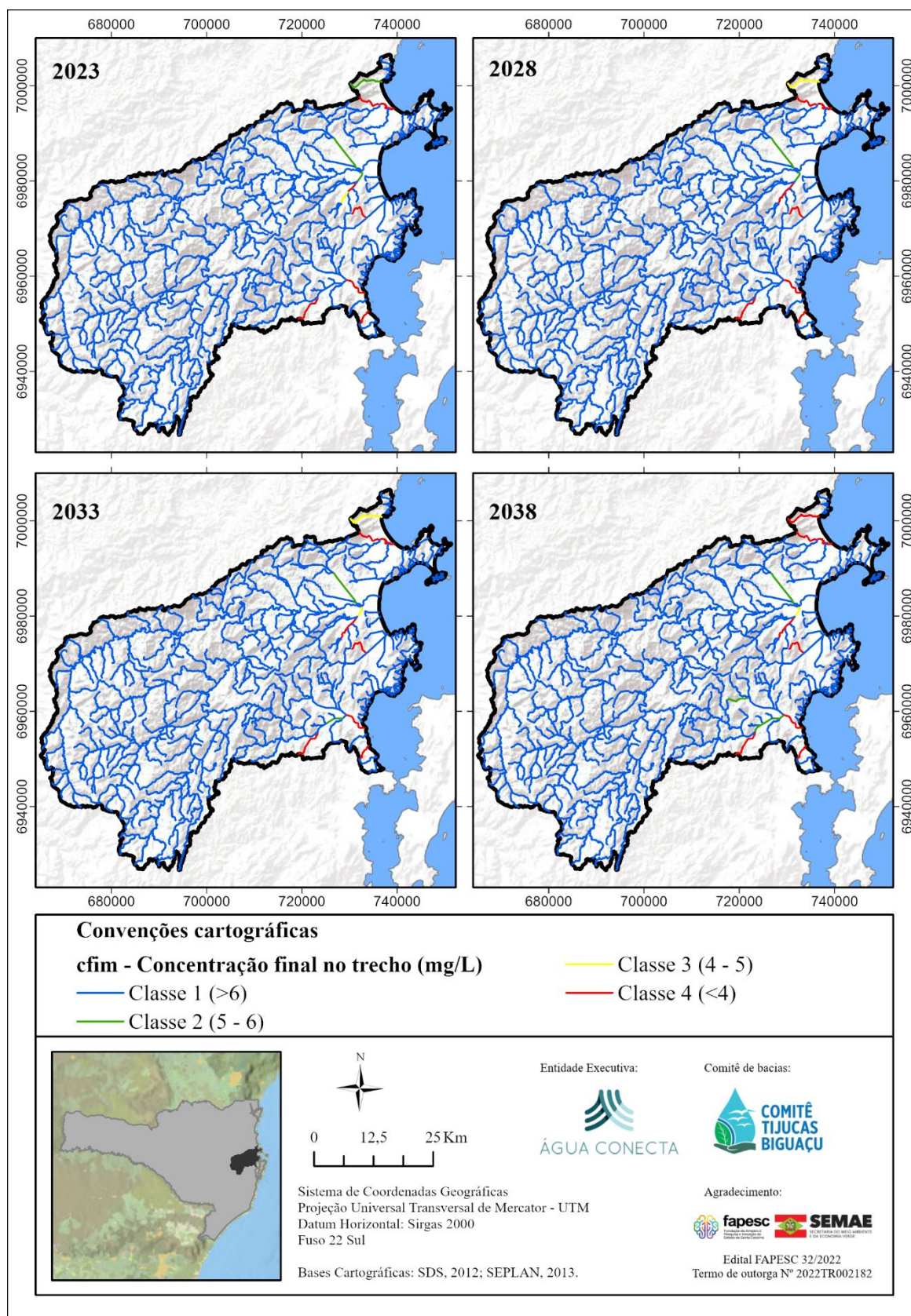
Figura 59 – Cenário atual (2023) e tendencial para os horizontes curto (2028), médio (2033) e longo (2038) prazo para a OD, dezembro (Tijucas) e janeiro (Biguaçu) de 2023.
