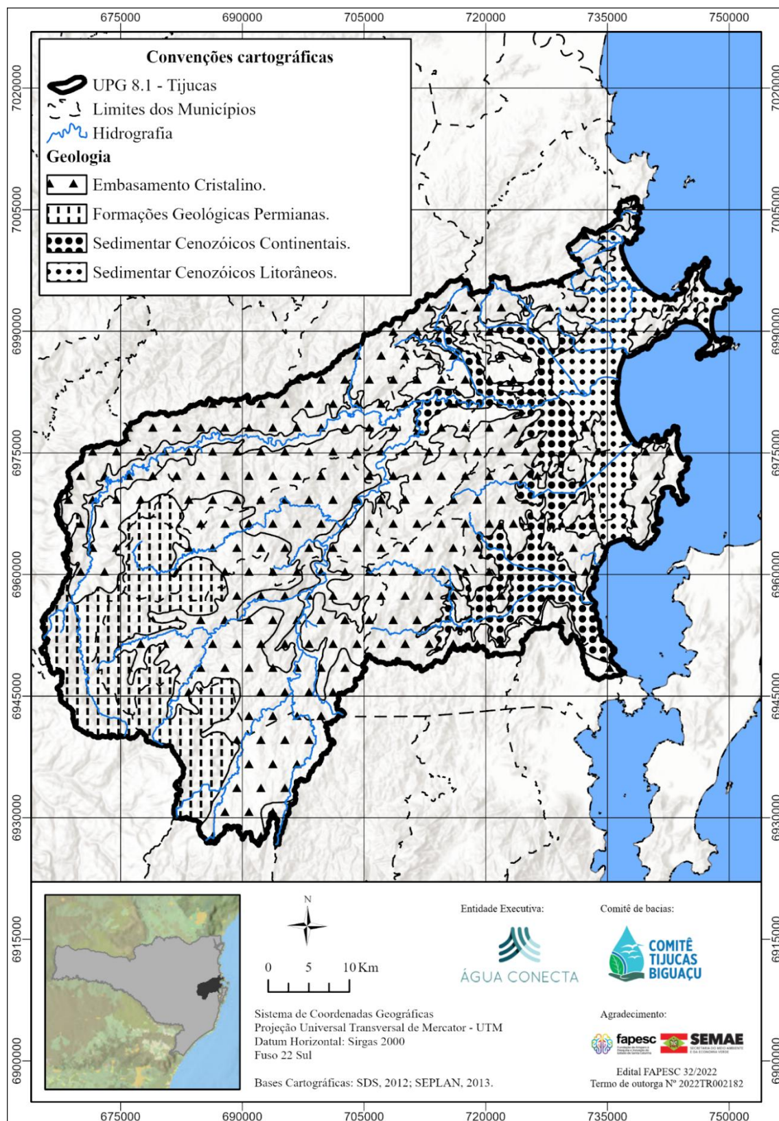
Figura 10 - Distribuição espacial das unidades hidroestratigráficas na UPG 8.1 - Tijucas, Biguaçu e bacias contíguas
