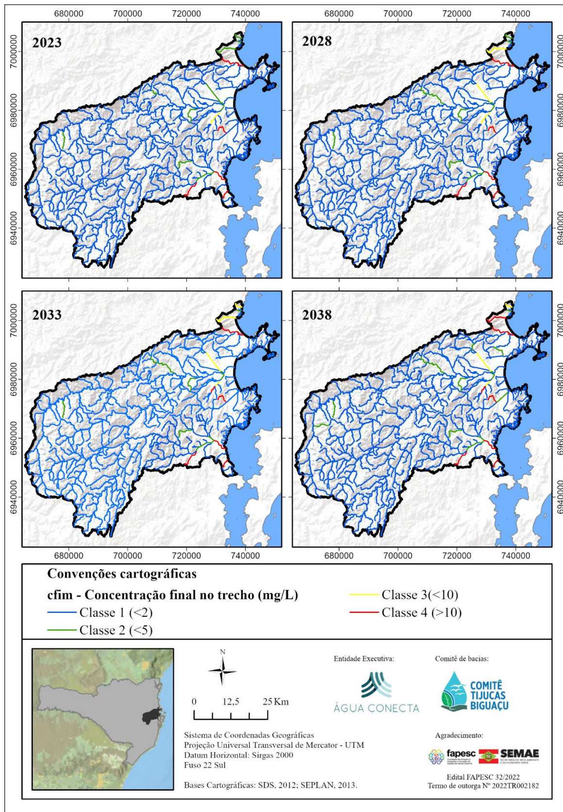
Figura 57 – Cenário atual (2023) e crítico para os horizontes curto (2028), médio (2033) e longo (2038) prazo para a DBO 5,20 , dezembro (Tijucas) e janeiro (Biguaçu) de 2023.
