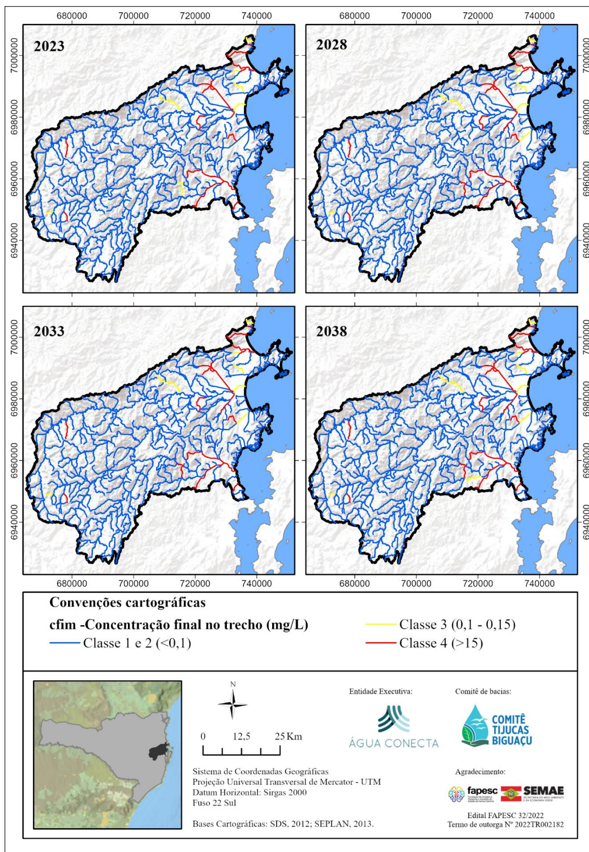
Figura 64 – Cenário atual (2023) e otimista para os horizontes curto (2028), médio (2033) e longo (2038) prazo para a Pt, dezembro (Tijucas) e janeiro (Biguaçu) de 2023.
