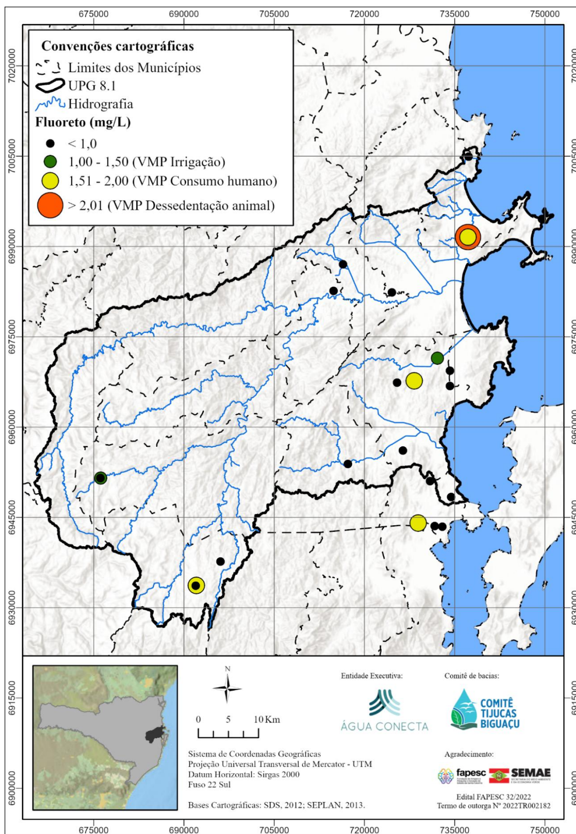
Figura 41 - Distribuição da concentração de fluoreto nas águas subterrâneas da UPG 8.1 – Tijucas
