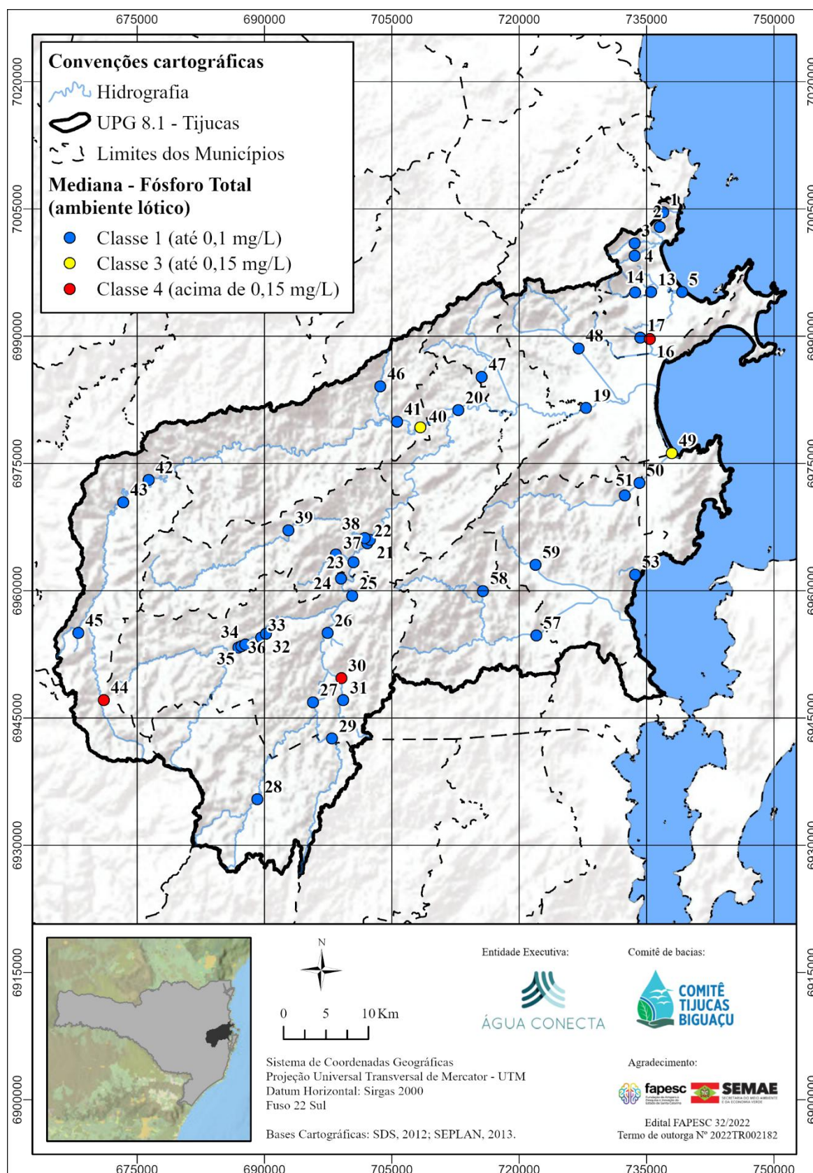
Figura 27 - Síntese dos dados da situação atual de fósforo total (Pt) na UPG 8.1 – Tijucas
